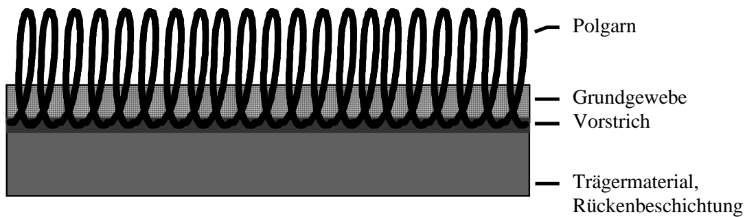
Abb. 7: Teppichquerschnitt
