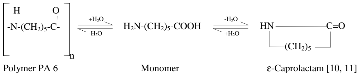
Abb. 13: Reaktionsgleichung zur Polymerisation/Depolymerisation von PA6 bzw. \epsilon -Caprolactam
