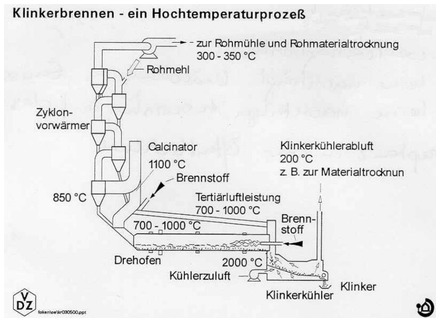
Abb. 25: Brennstoffaufgabe des EBS beim Klinkerbrennen [22]
