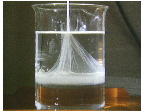
Abb. 17: Polymerisation von PA [13]
