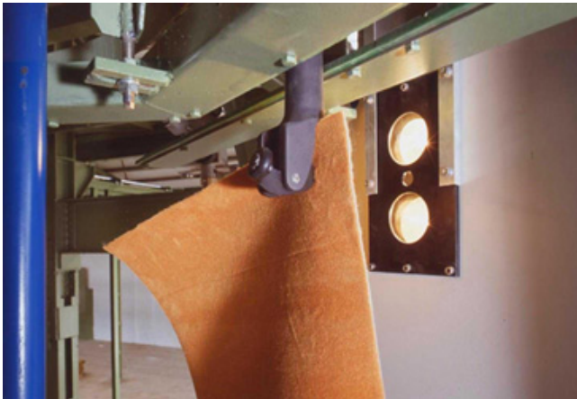
Abb. 11: CarRID™ (Prototyp) (li.) und Sortierklammern (re.) [ 8,9]
