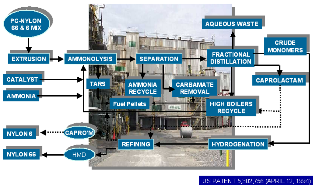
Abb. 19: Recyclingverfahren DuPont [15]
