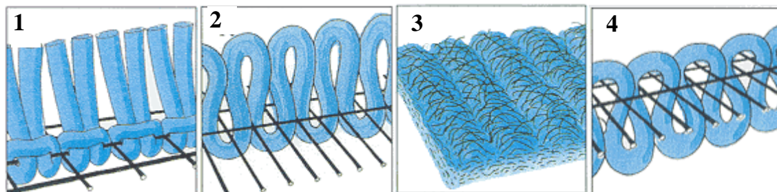
Abb. 6: Herstellarten von Teppichen Geknüpfter (1), gewebter (2), genadelter (3) und getufteter (4) Teppich
