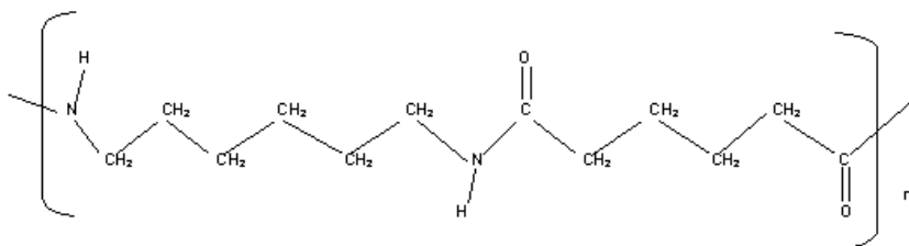
Abb. 15: Strukturformel PA 66
