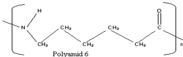
Abb. 14: Strukturformel PA 6
