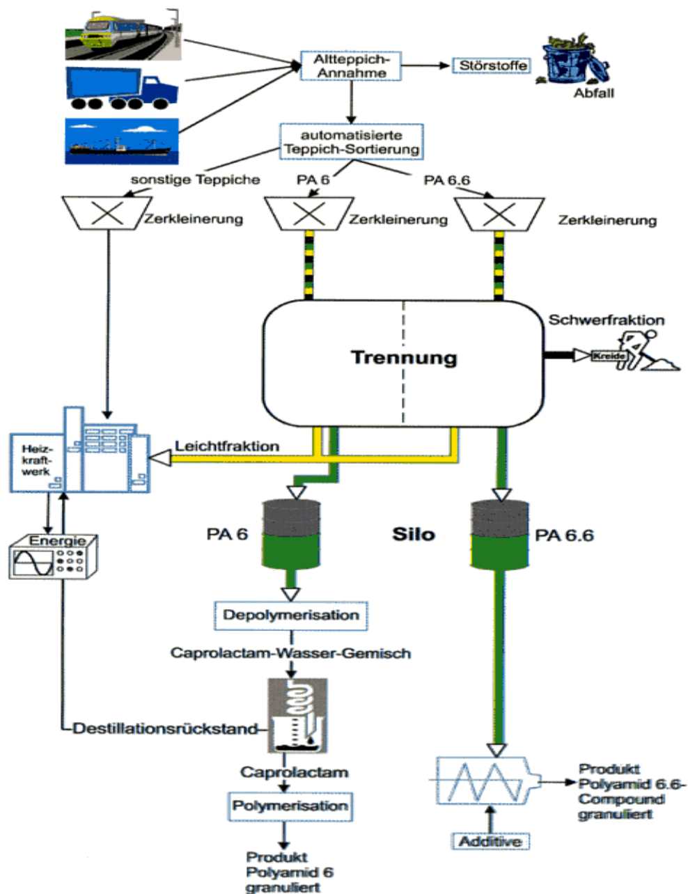
Abb. 16: Fließbild der Anlage der Polyamid 2000 AG [12]
