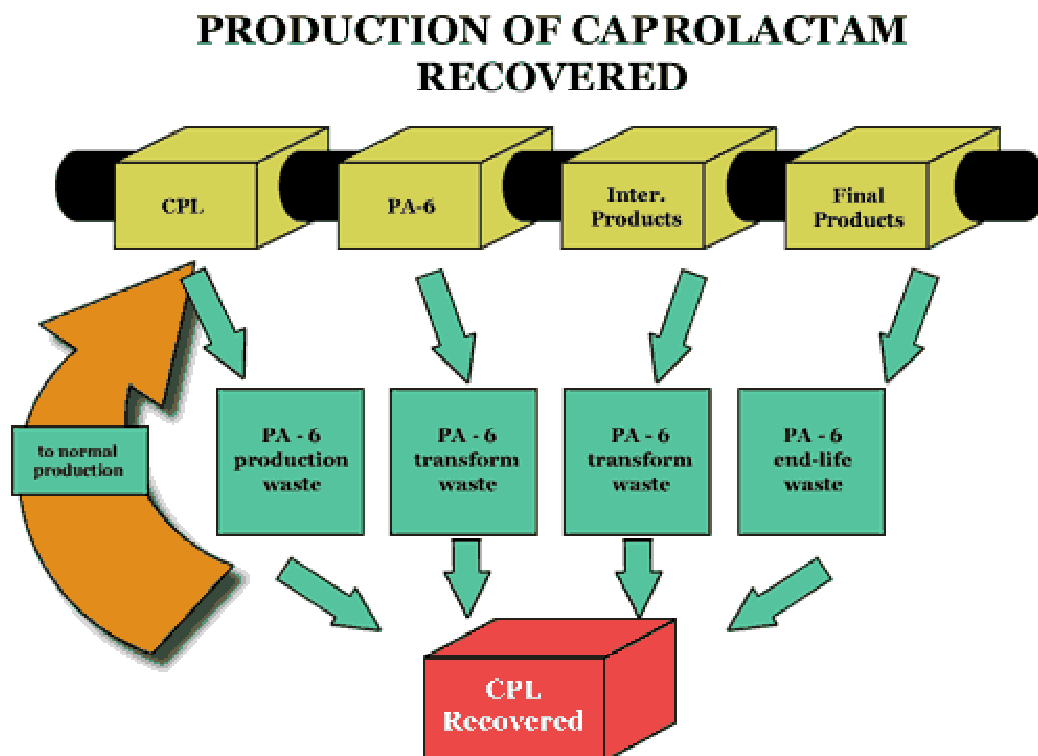
Abb. 20: Einsatz von Produktionsabfällen in der PA 6-Produktion (CPL= Caprolactam) [17]
